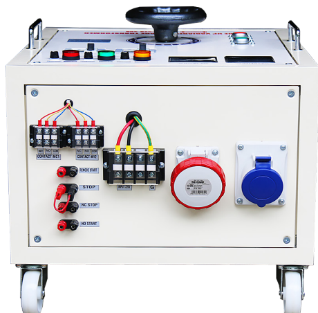
จุดต่อใช้งานด้านหลัง VARIAC
